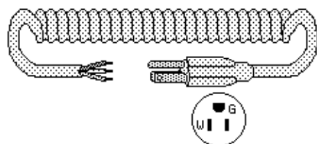
NEMA 5-15P
